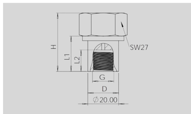
NPT 内螺纹
