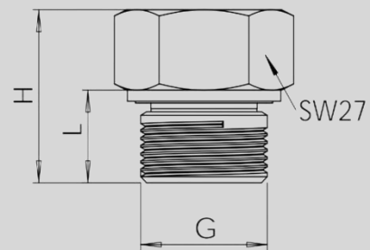
直螺纹
